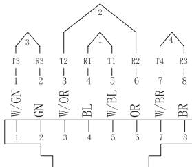
T568A
