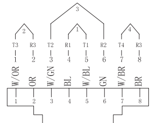
T568B
